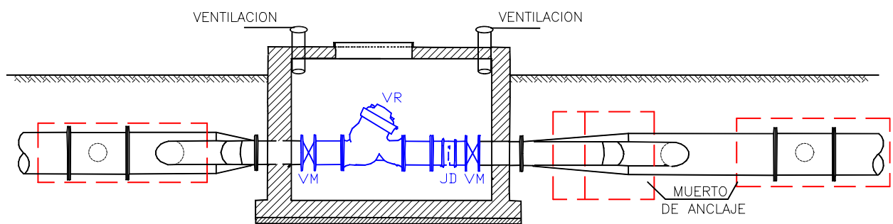
Figura 9 Cámara para Válvula de Control
