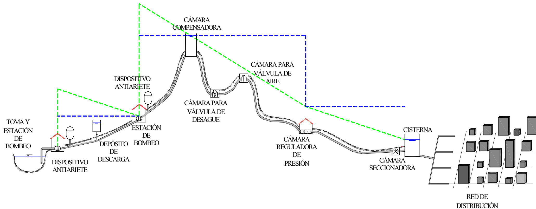
Figura 1 Componentes Principales de un Acueducto a Presión
