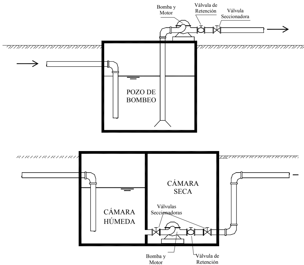
Figura 3 Estaciones de Bombeo con Cámara Seca
