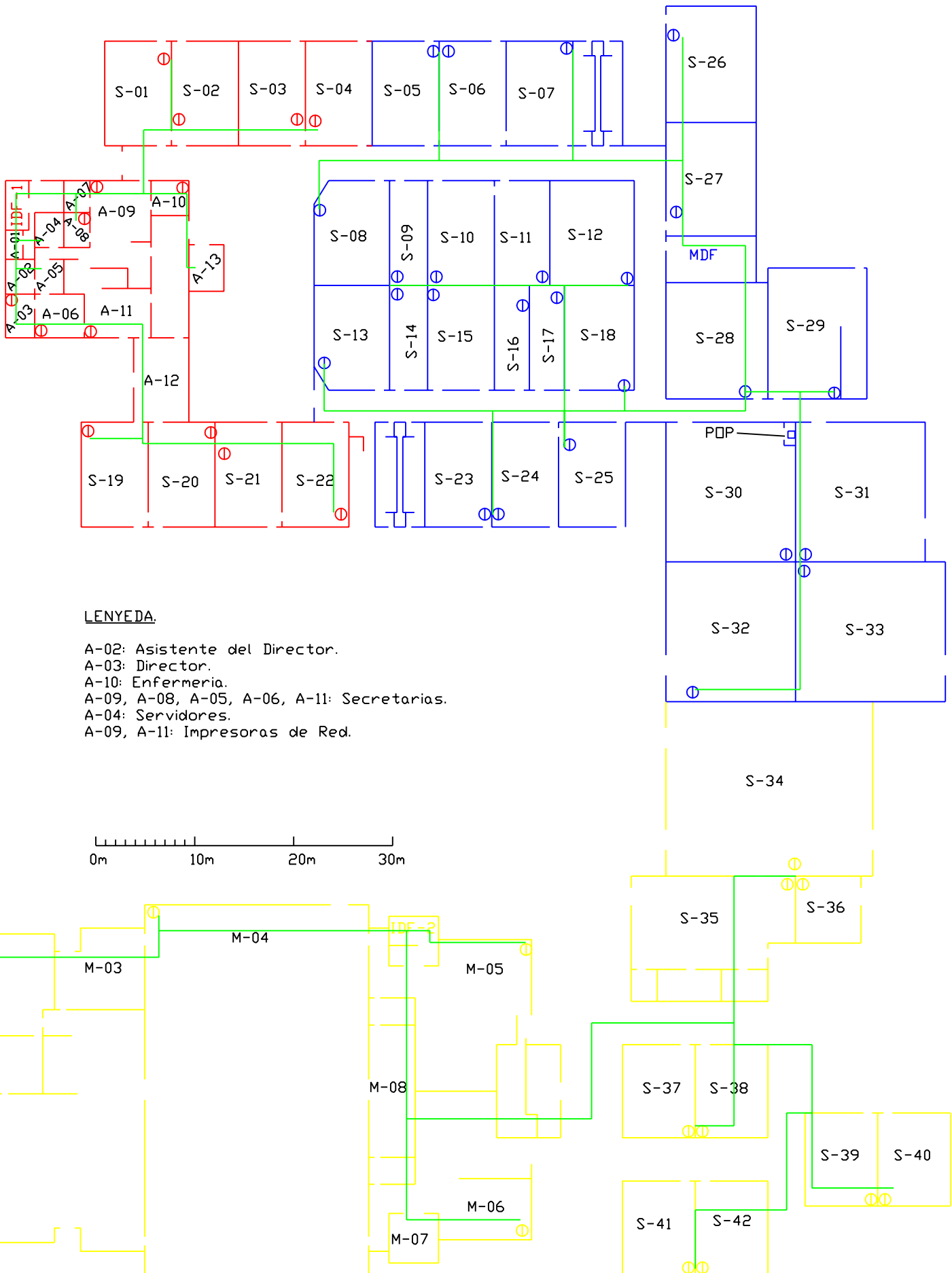
Anexo 5 - Mapa de canalización de cableado horizontal
