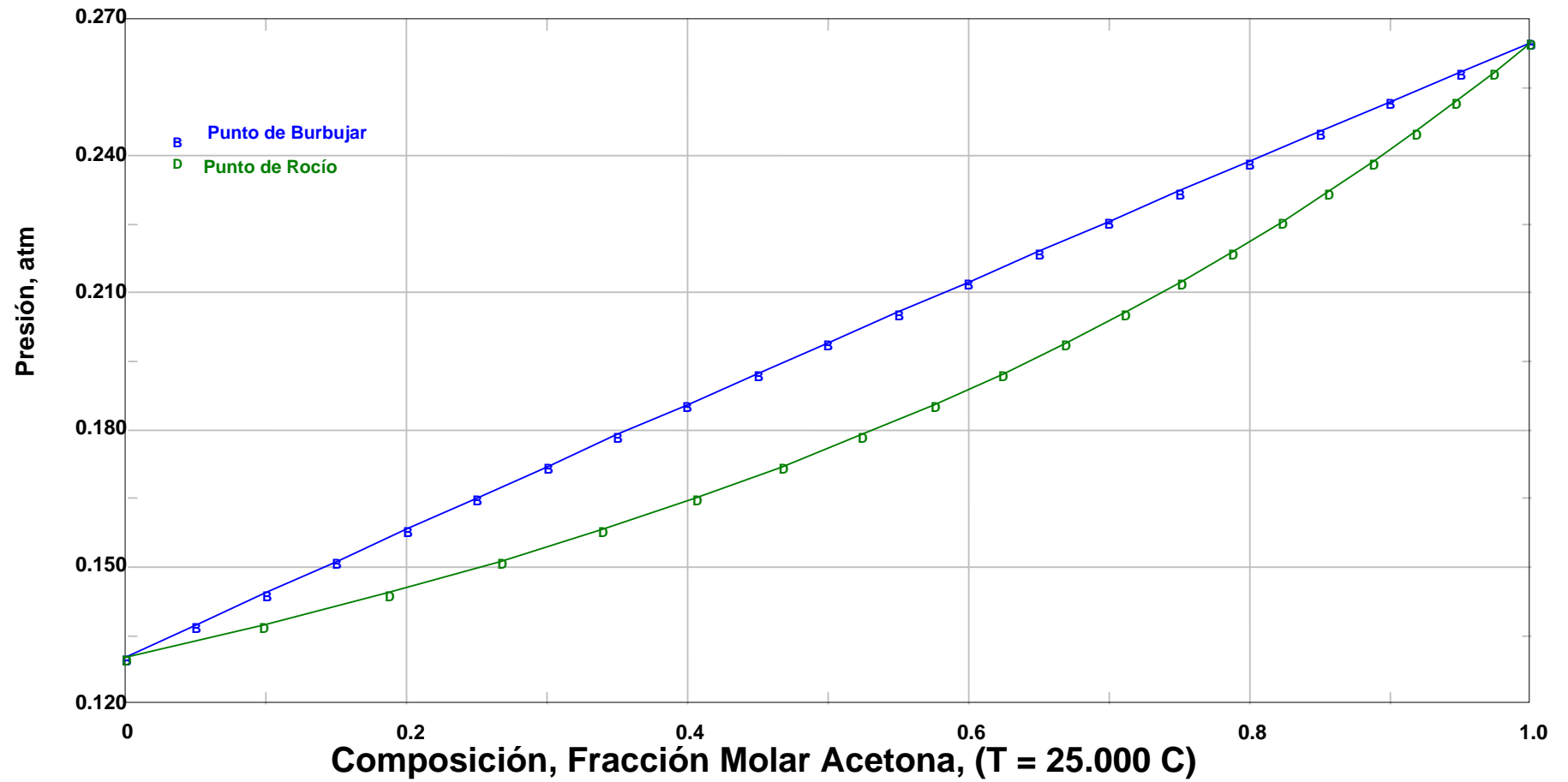
Figura N° 4: Diagrama P-X-Y para Acetona y Ciclohexano. Redlich-Kwong Soave.
