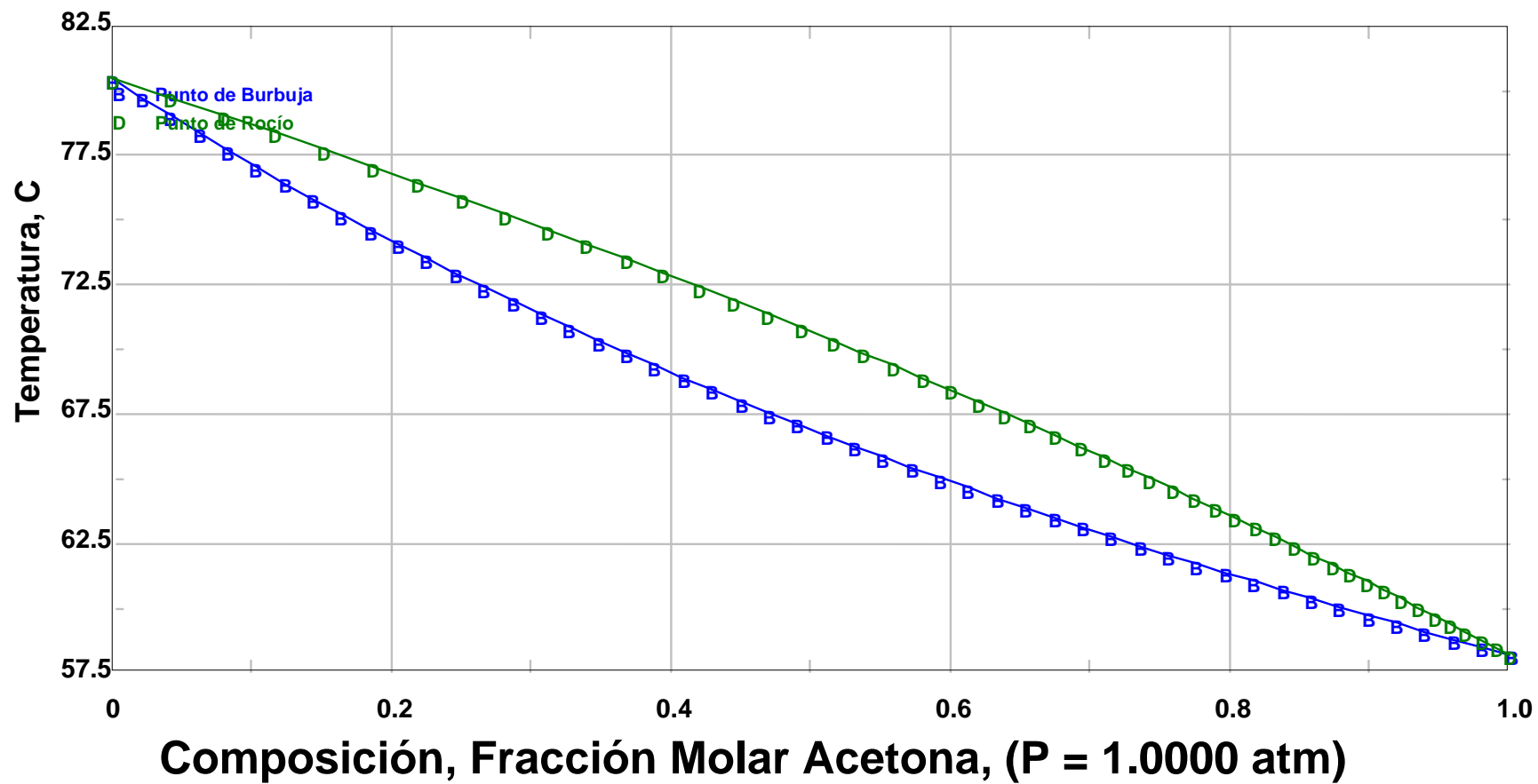
Figura N° 2: Diagrama T-X-Y para Acetona y Ciclohexano. Peng Robinson.
