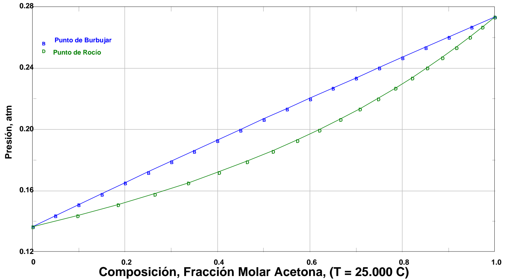
Figura N° 5: Diagrama P-X-Y para Acetona y Ciclohexano. Peng Robinson.
