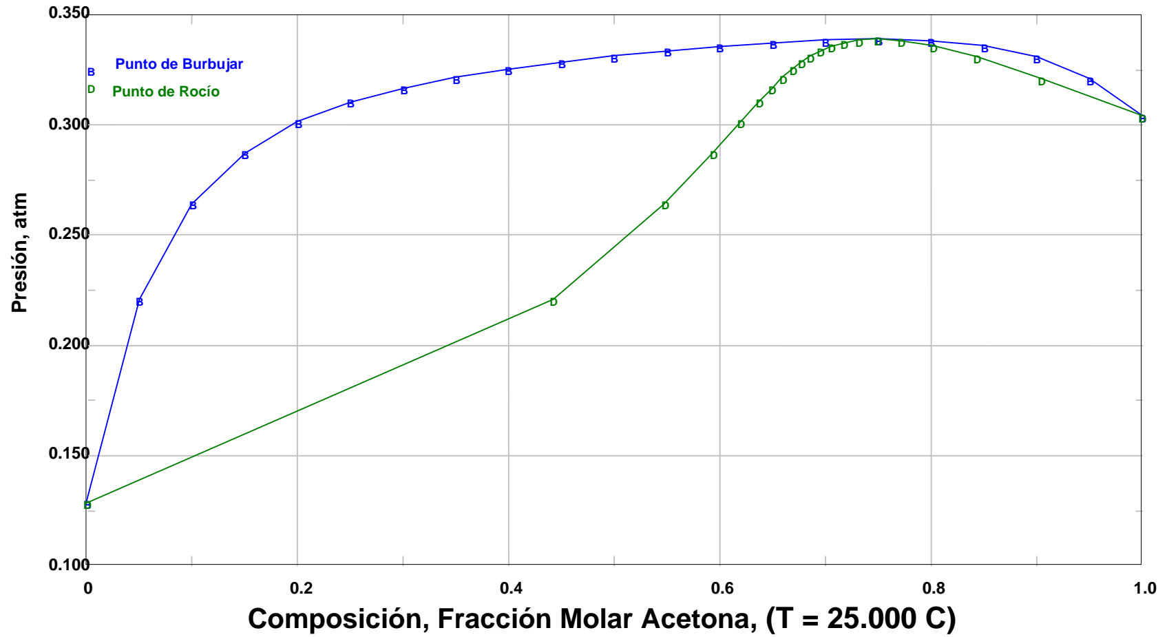
Figura N° 6: Diagrama P-X-Y para Acetona y Ciclohexano. Modelo de Wilson
