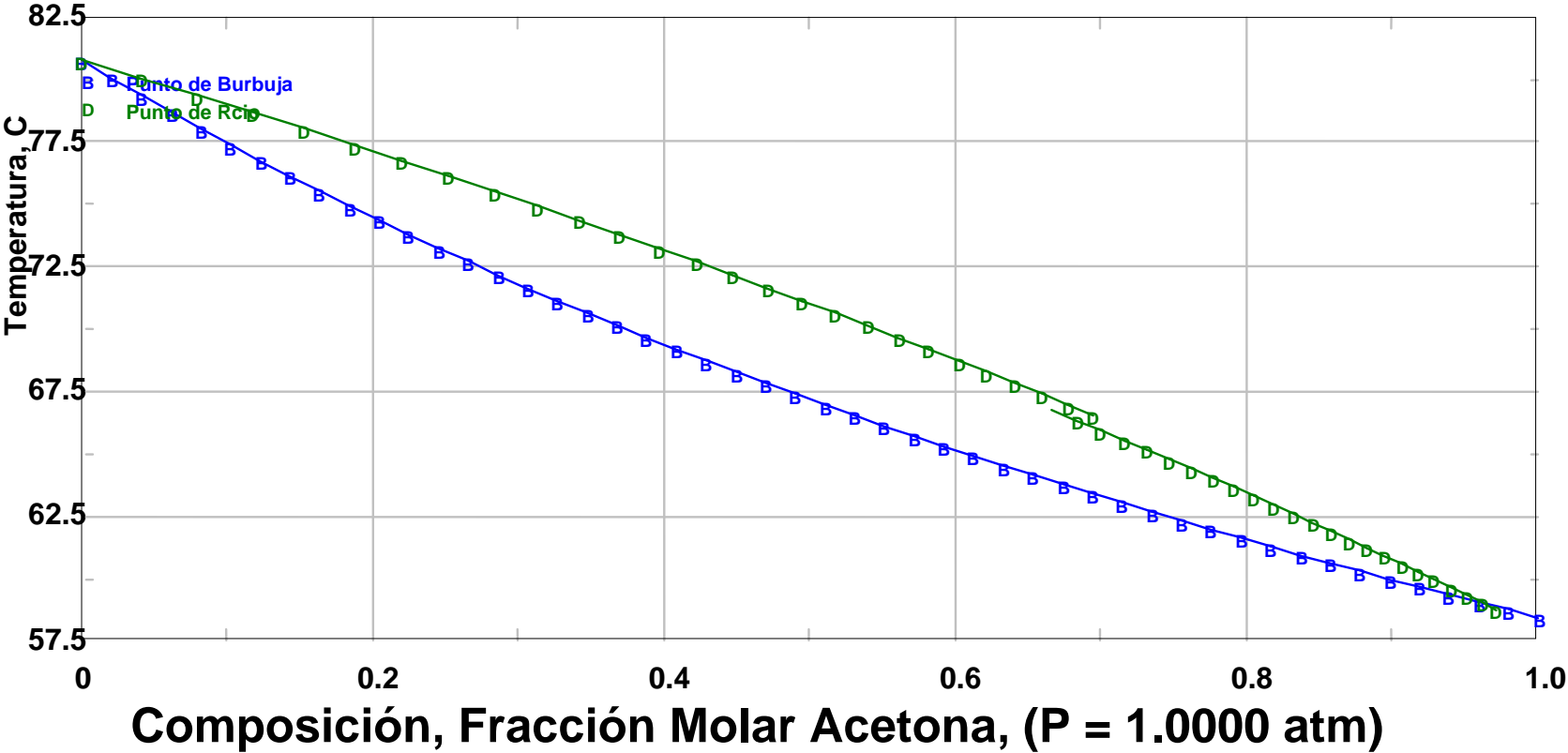
Figura N° 1: Diagrama T-X-Y para Acetona y Ciclohexano. Redlich-Kwong Soave.
