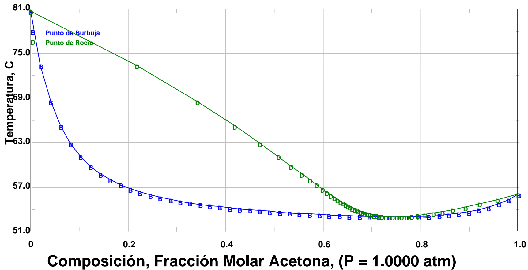
Figura N° 3: Diagrama T-X-Y para Acetona y Ciclohexano. Modelo de Wilson
