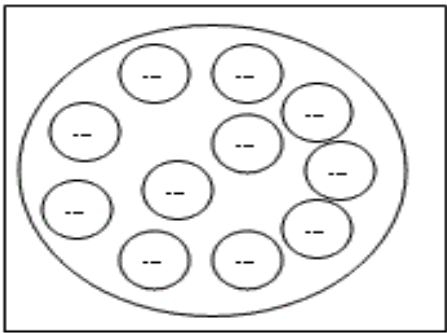
نموذج طومسون
