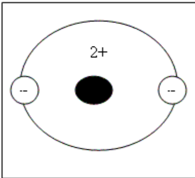
نموذج رذرفورد لذرة الهيليوم
