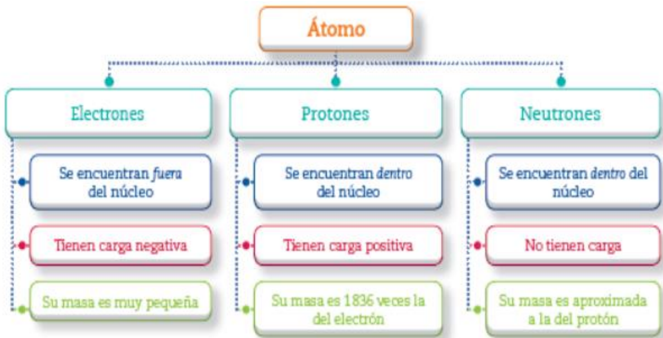
Diagrama 1.3 Características de las partículas elementales del átomo. ESTRUCTURA DEL NUCLEO
