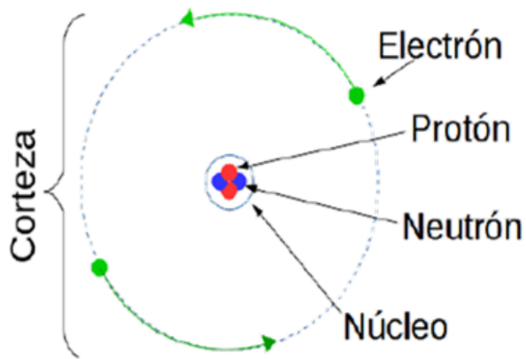
Diagrama 1.3 Características de las partículas elementales del átomo. ESTRUCTURA DEL NUCLEO
