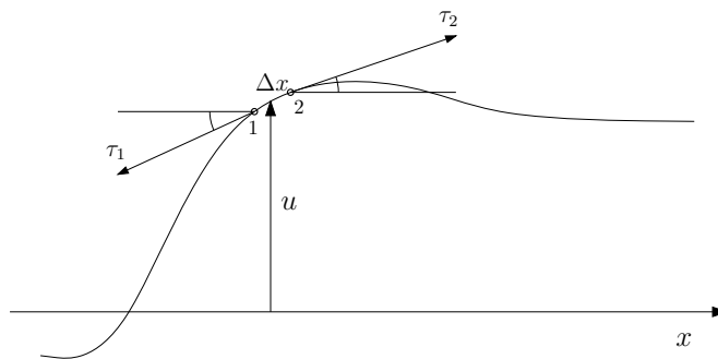
Figura 4.1: Sección transversal de la membrana deformada
