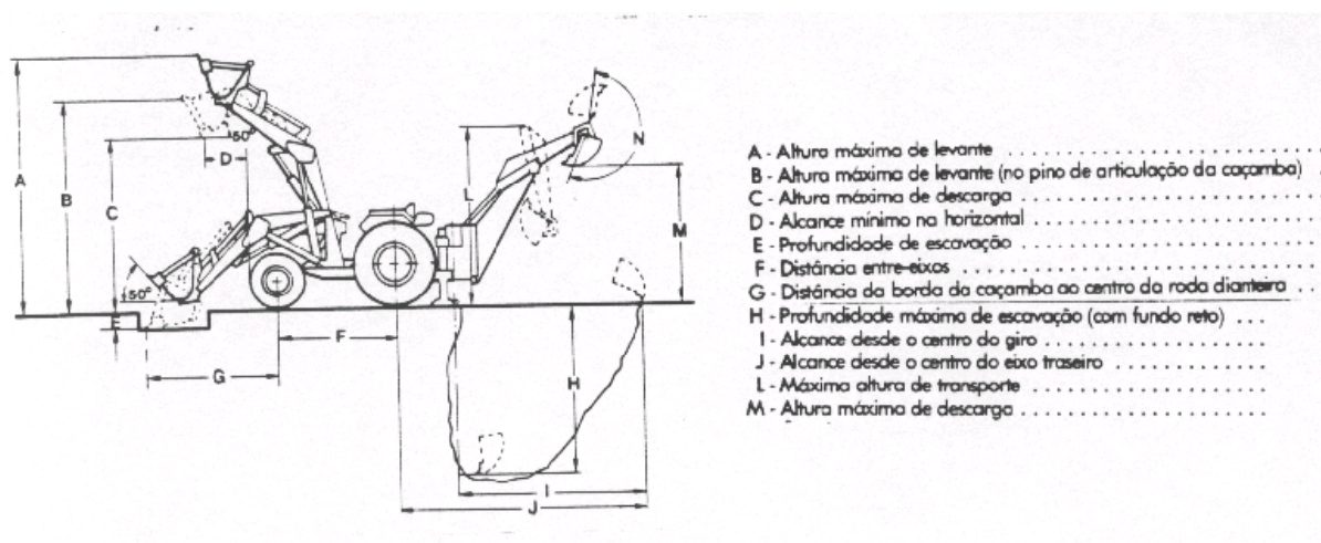
Figura 14 – Retro-escavadora equipada com pá-carregadora.
