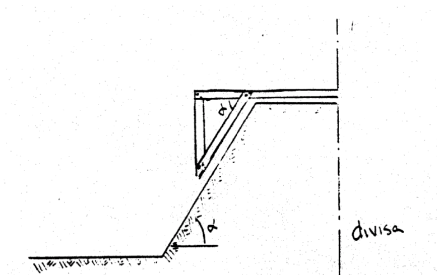
Figura 5 – Gabarito para controle de inclinação de taludes.
