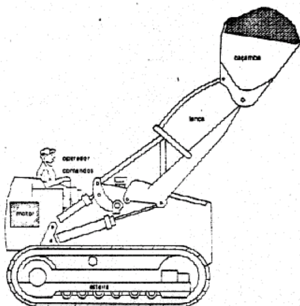
Figura 6 – Pá carregadora.
