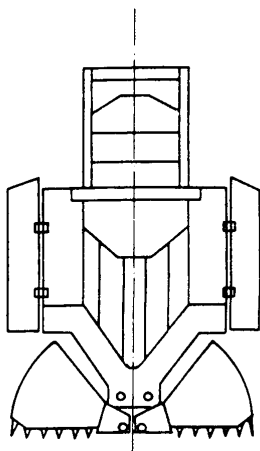
Figura 3.19: Clam-shell
