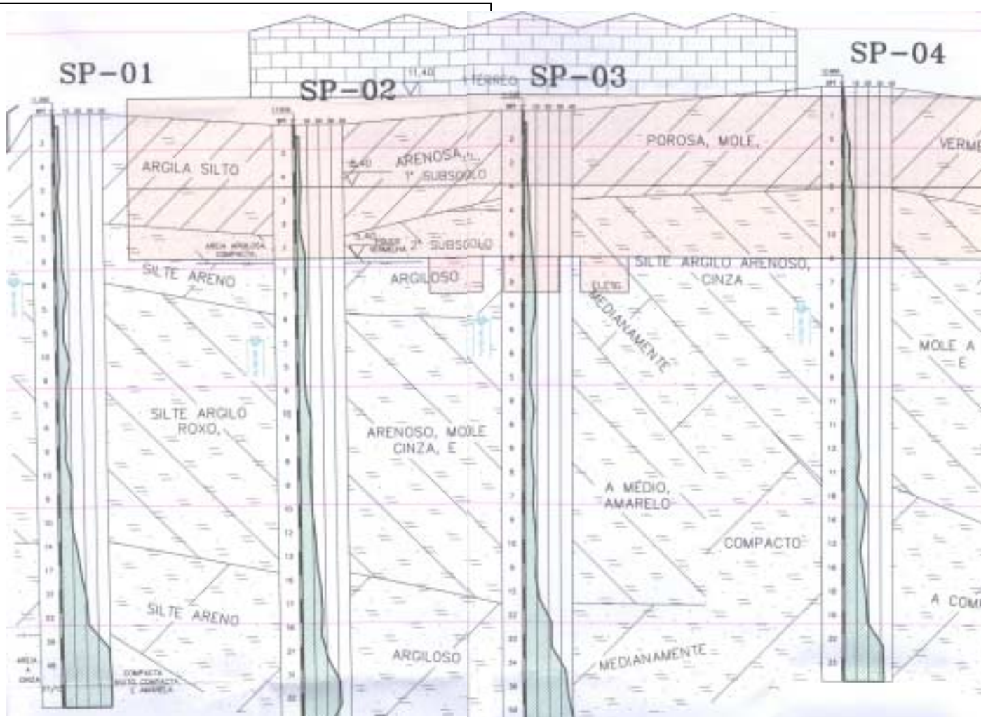
Figura 2.2 – Perfil do terreno, a partir da avaliação por sondagem à percussão.
