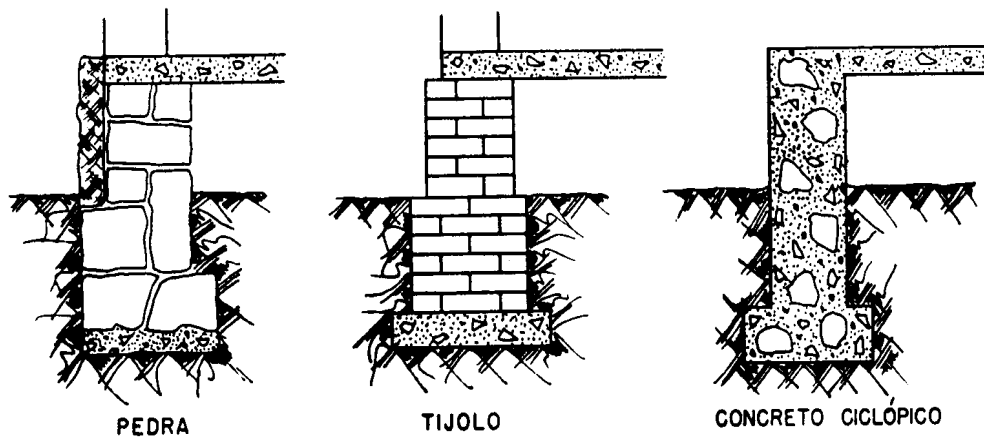
Figura 3.2: Tipos de alicerce
