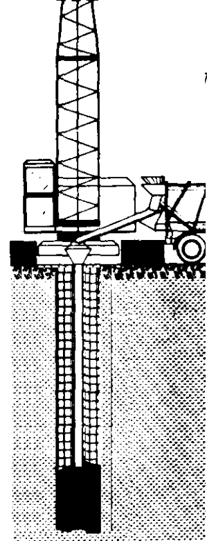
Figura 3.18: Concretagem submersa
