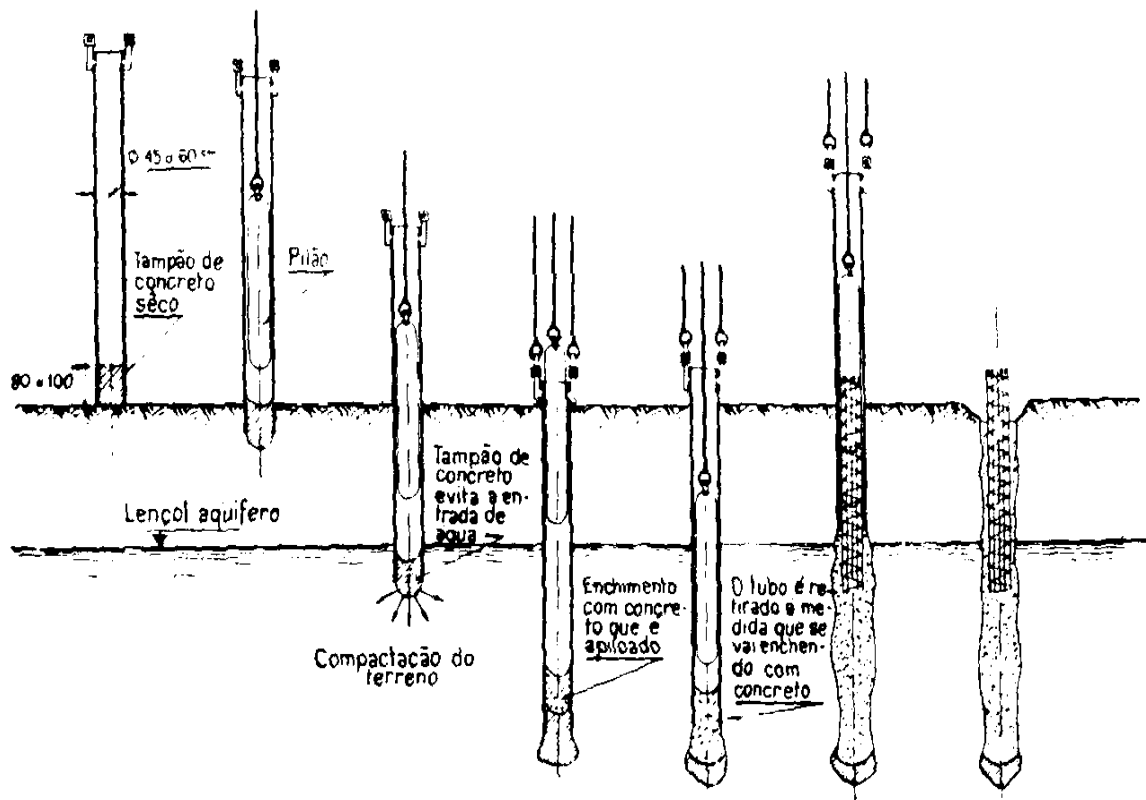
3.14: Estaca Franki
