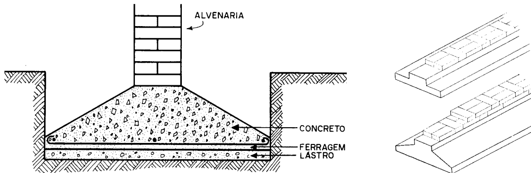
Figura 3.5: Sapata corrida
