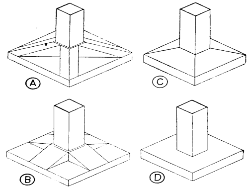
Figura 3.4: Sapatas isoladas
