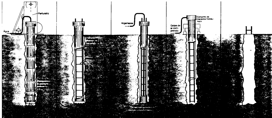
Figura 3.15: Estaca raiz
