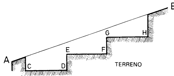
Figura 3.3: Execução do alicerce em declive
