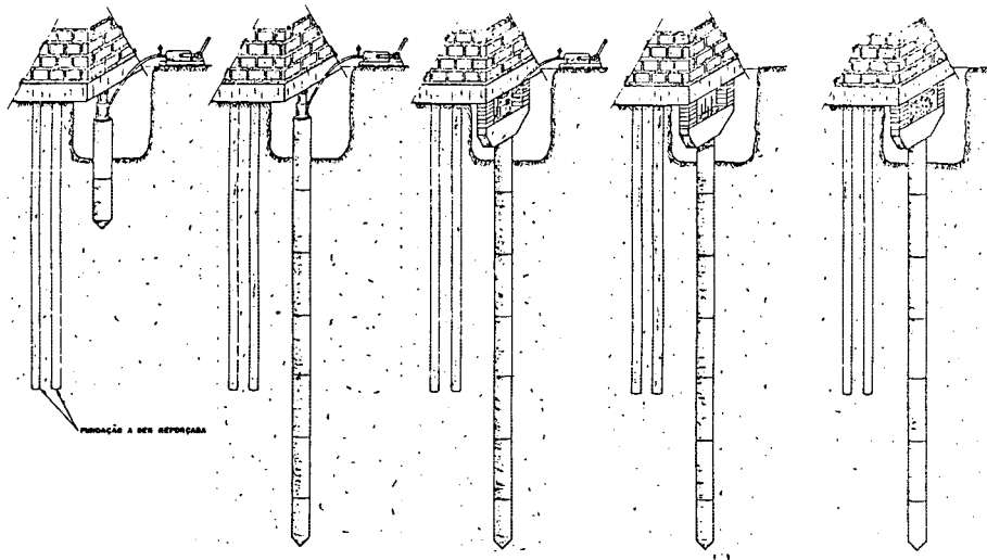
Figura 3.12: Estaca Mega
