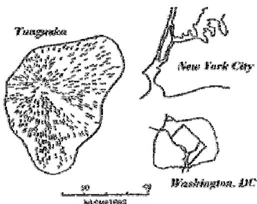
Rys. Kształt Eksplozji tunguskiej oraz porównanie do Nowego Jorku i Waszyngtonu.
