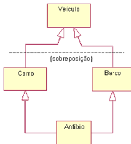
Representação de uma Generalização de Sobreposição
