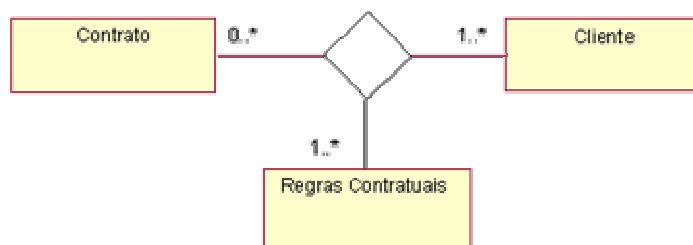
Representação de uma Associação Ternária
