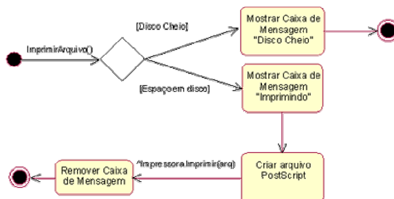
Representação de um Diagrama de Atividades de um servidor de impressão
