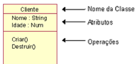
Representação de uma Classe
