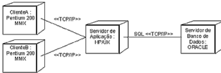
Representação de um Diagrama de Execução de Associação entre Nodes
