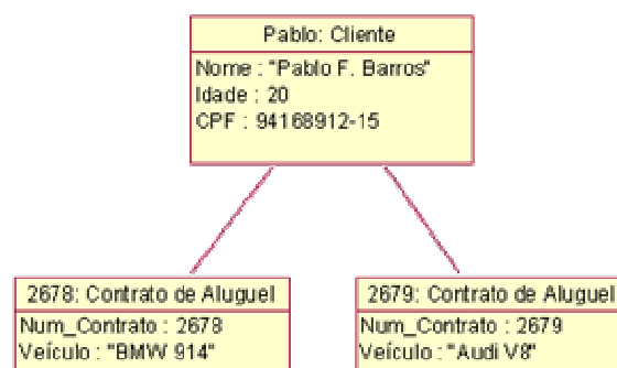
Representação de um Diagrama de Objetos onde a classe Cliente se relaciona de 1 para n com Contrato de Aluguel, por isso um Objeto da Classe Cliente pode ter um ou vários contratos.
