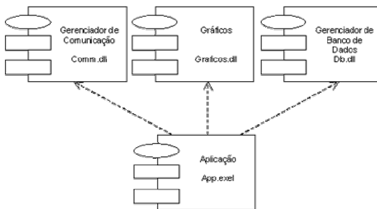
Representação de um Diagrama de Componentes
