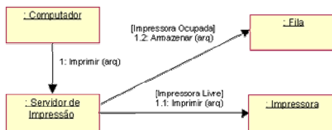
Representação de um Diagrama de Colaboração de um servidor de impressão
