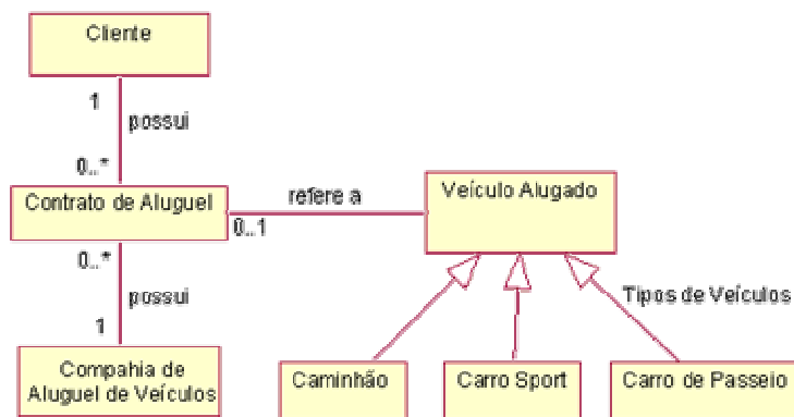
Representação através de Diagrama de Classe de uma empresa de aluguel de veículos
