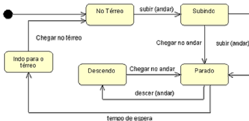
Representação do Diagrama de Estados de um elevador
