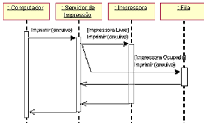
Representação de um Diagrama de Sequência de um servidor de impressão
