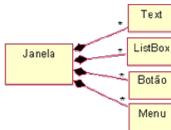
Representação de uma Agregação de Composição
